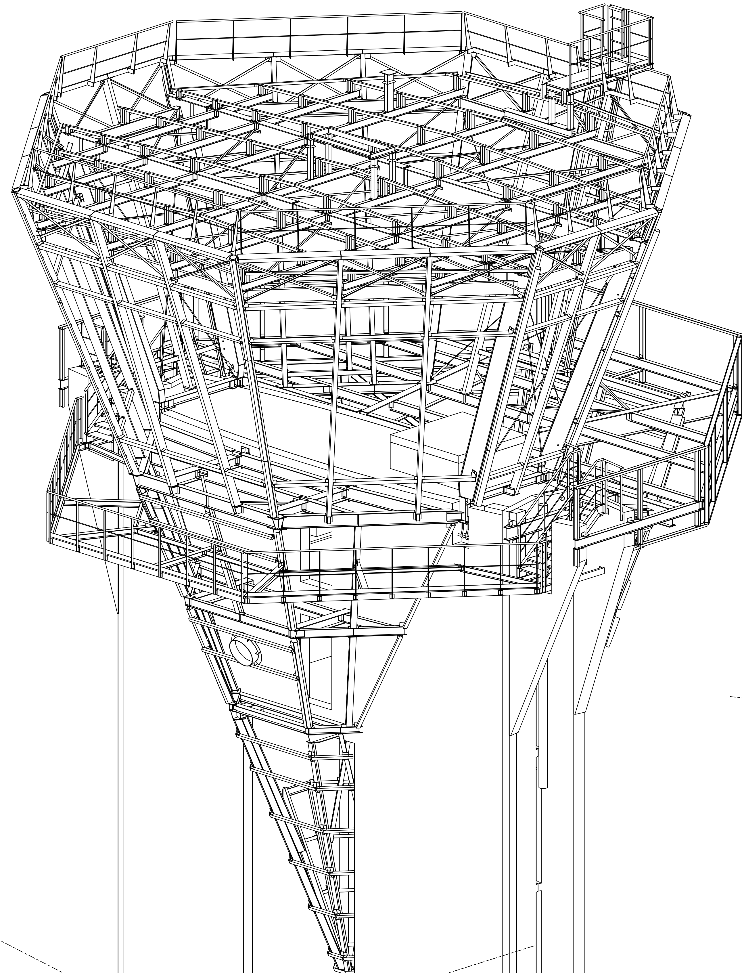
PERSPECTIVE AVANT - (COTE PISTE)
