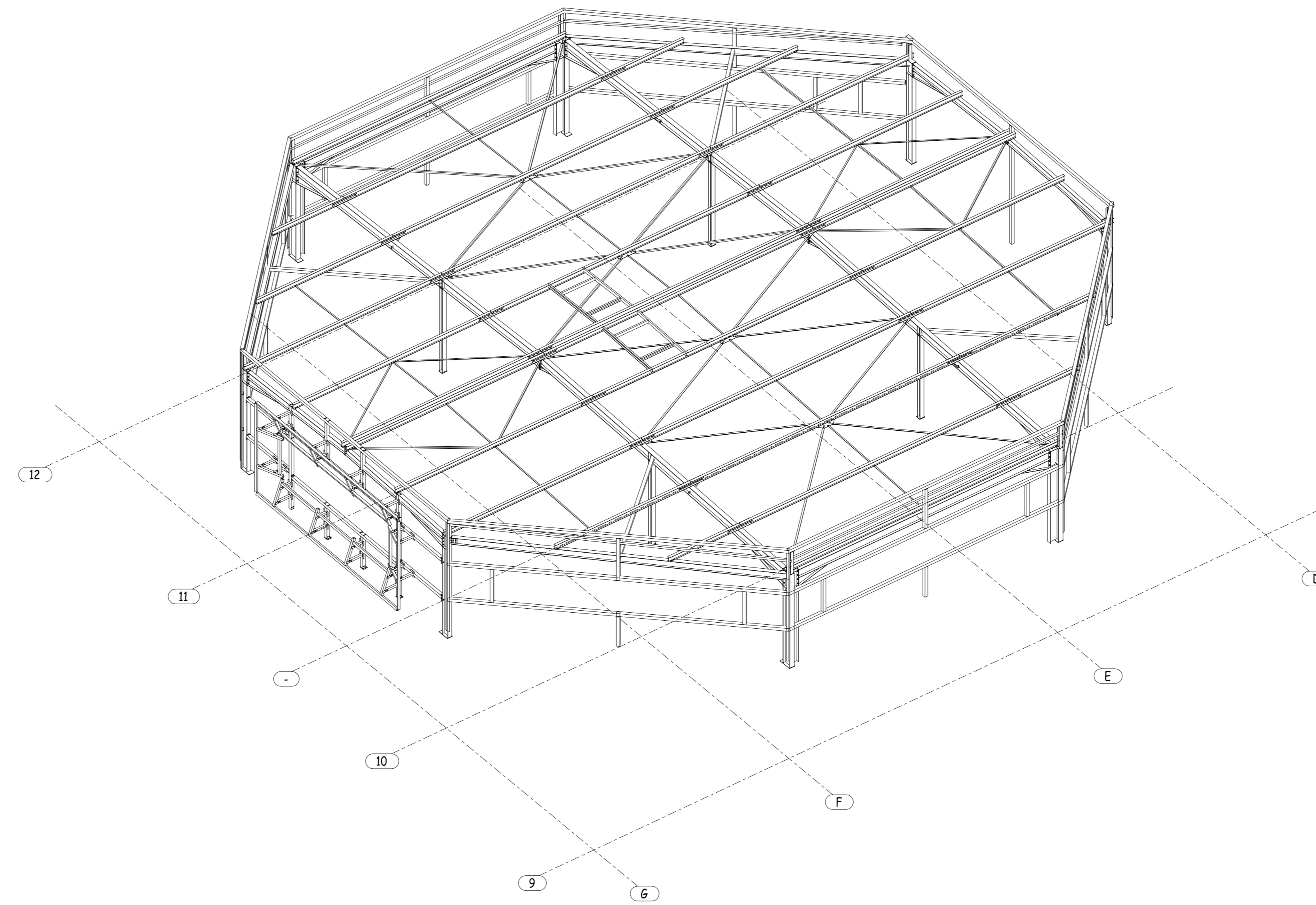
CHARPENTE R+1 SEULE VUE EST
