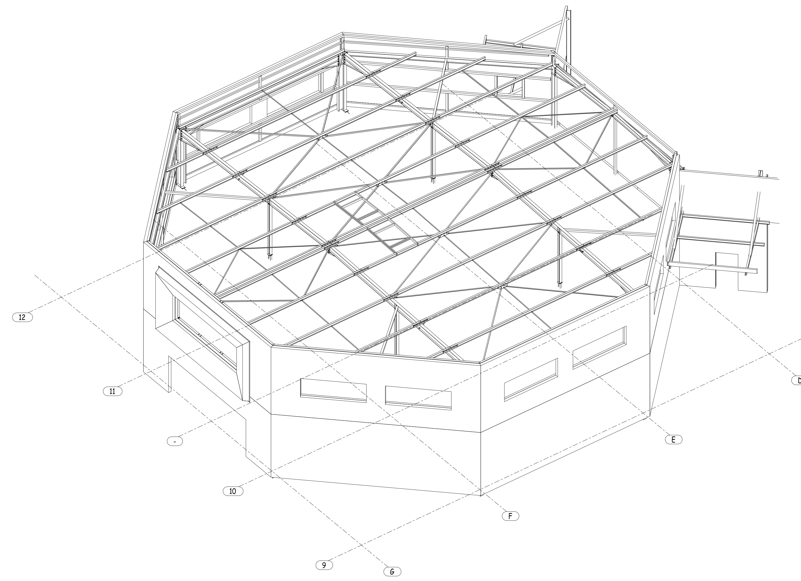
PERSPECTIVE DE L'ENSEMBLE VUE EST
