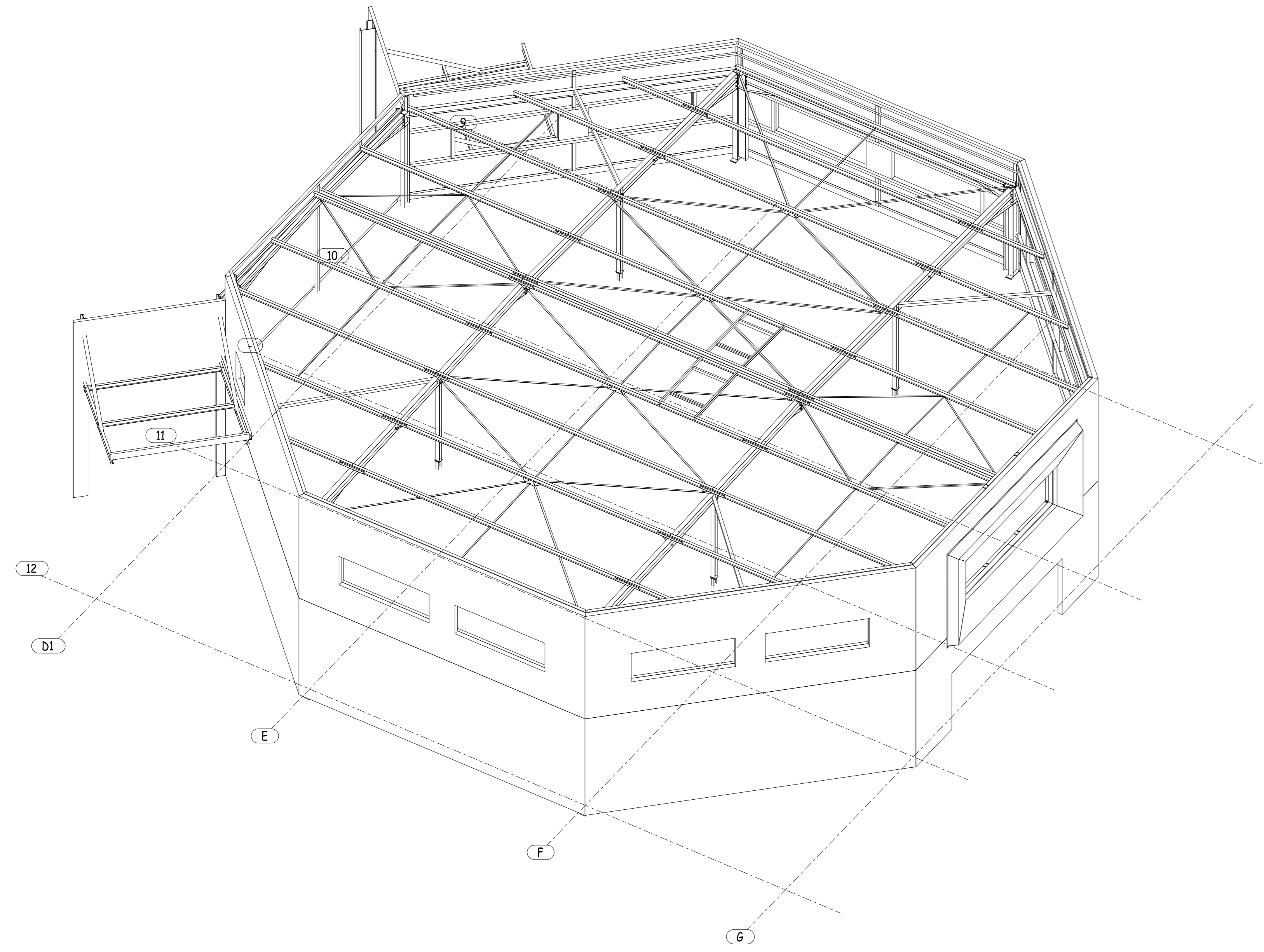
PERSPECTIVE DE L'ENSEMBLE VUE OUEST
