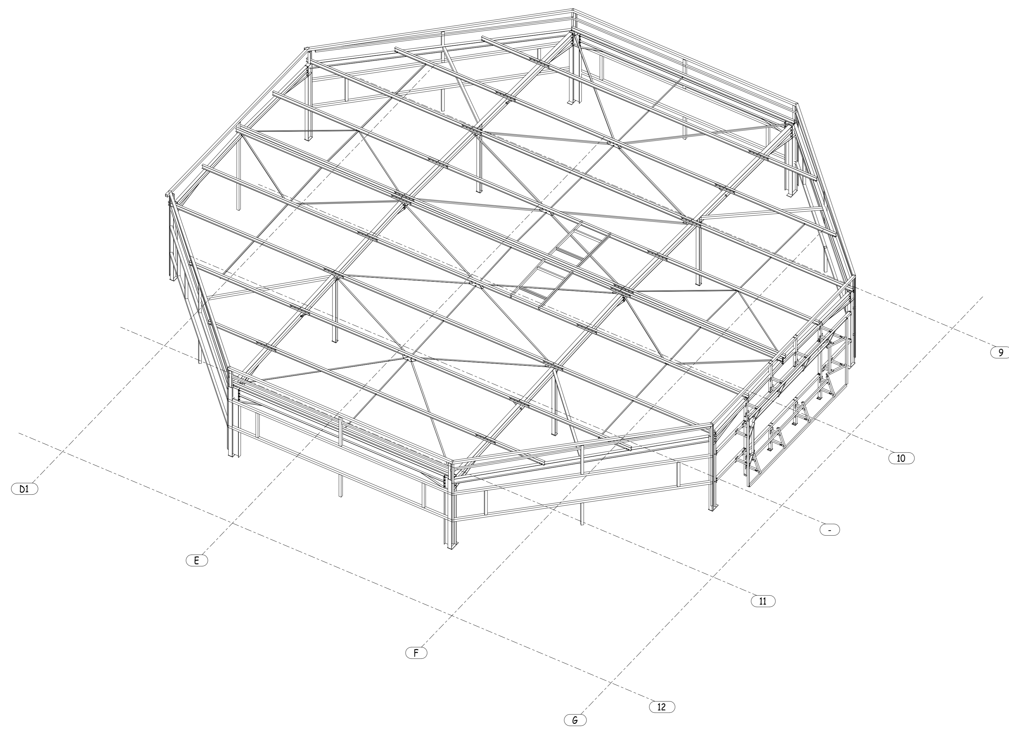
CHARPENTE R+1 SEULE VUE OUEST
